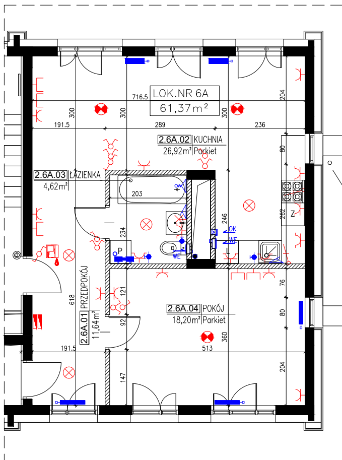
Rzut lokalu 1:100
